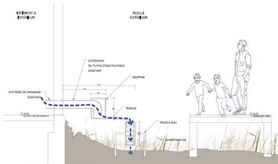
Coupe schématique installation de la roue à eau
